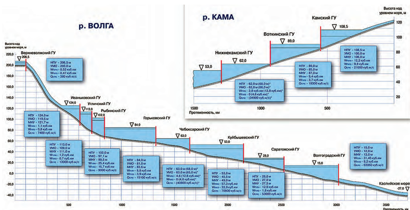
Рис. 1.23. Схема Волжско-Камского каскада водохранилищ (по данным Росводресурсов)
