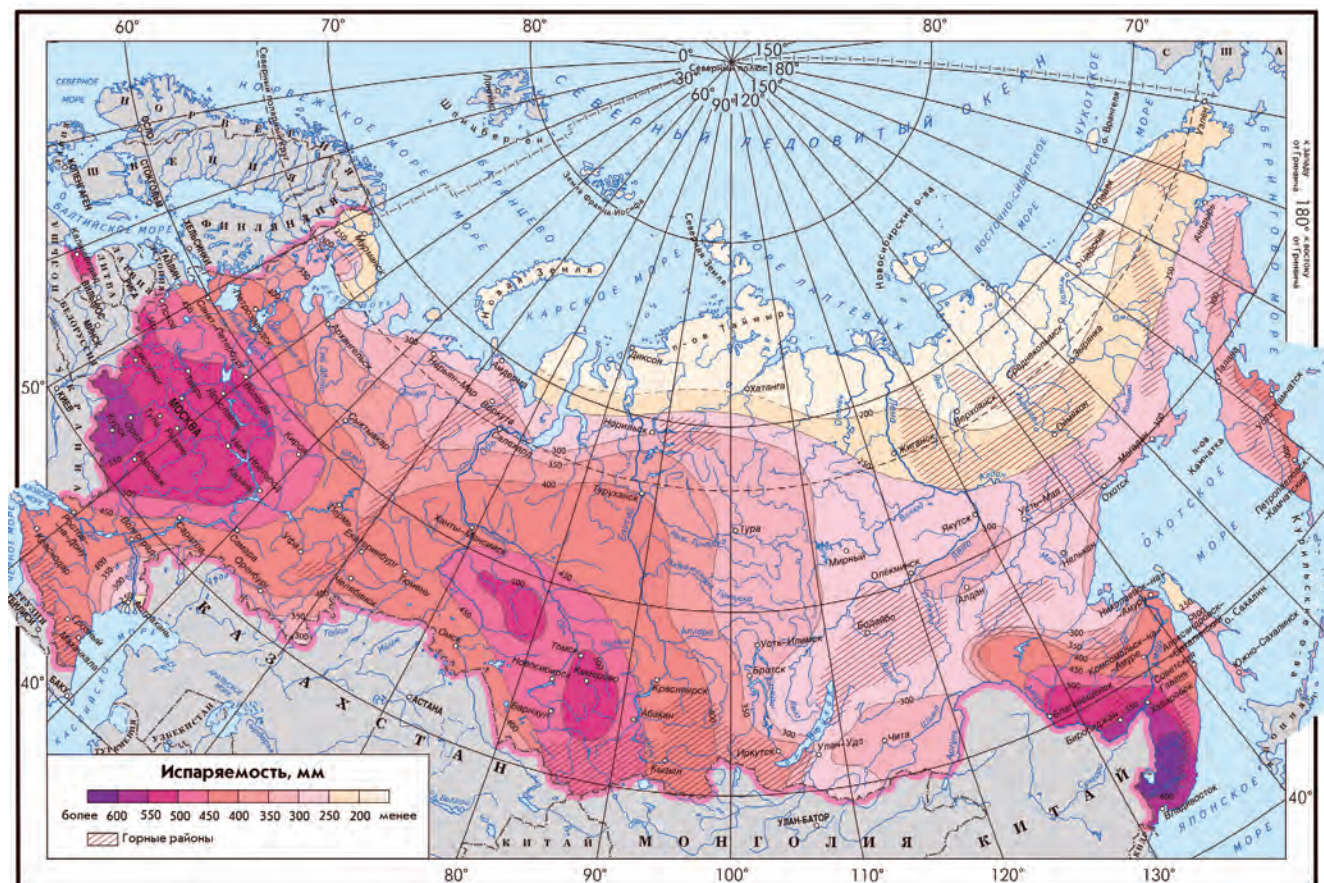
Рис. 1.5. Распределение фактического испарения с поверхности суши России, мм
