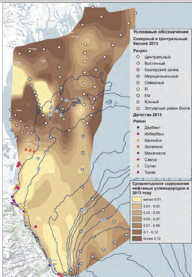
Рис. 1.25. Распределение нефтяных углеводородов в водах Северного и Центрального Каспия в 2013 г., мг/дм 3
