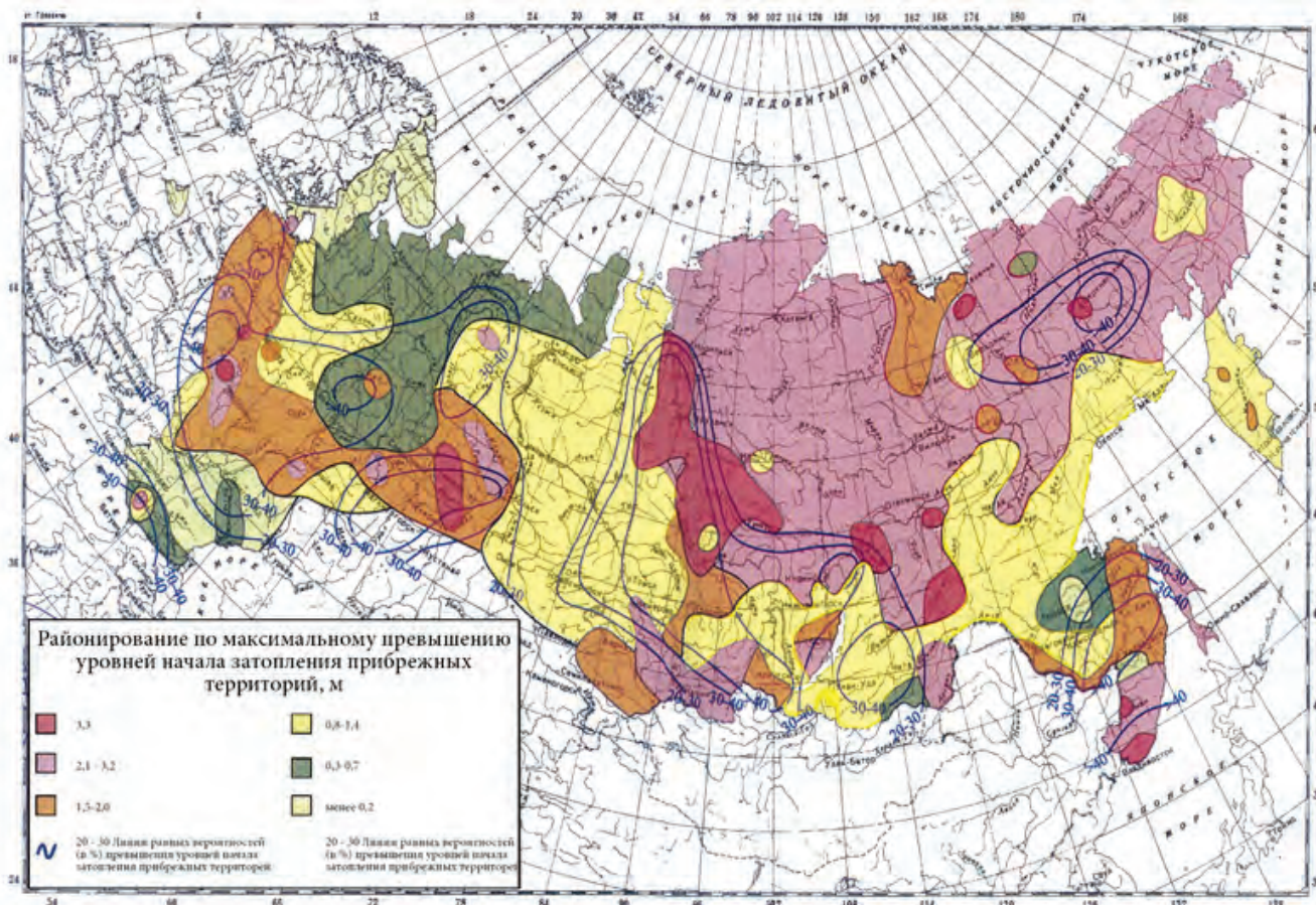
Рис. 3.7. Районирование территории России по степени опасности наводнений
