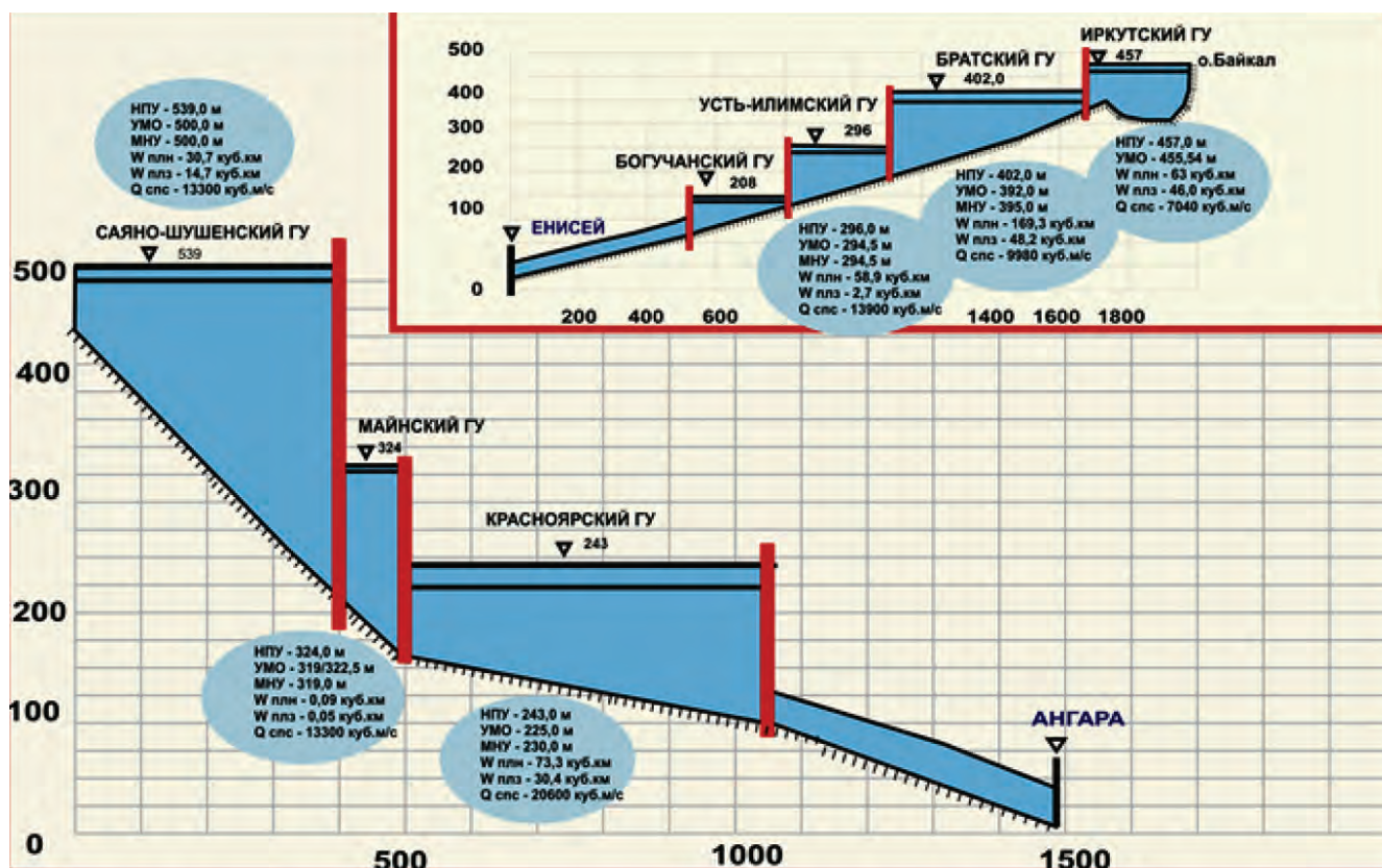
Рис. 1.24. Схема Ангаро-Енисейского каскада водохранилищ (по данным Росводресурсов)
