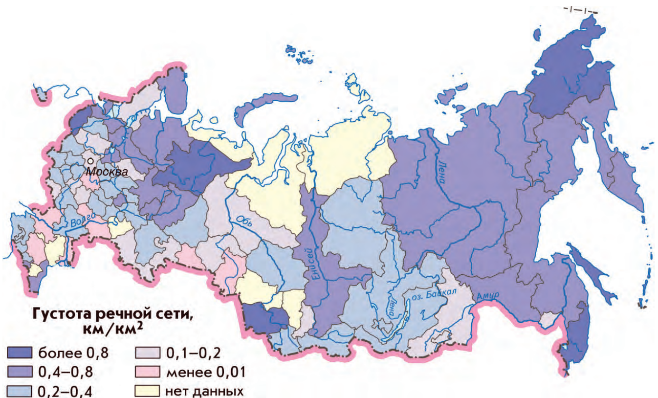
Рис. 1.7. Густота речной сети в России
