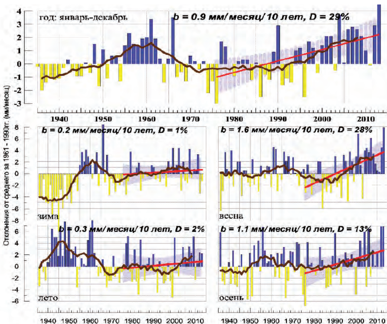
Рис. 1.3. Средние за год аномалии сезонных сумм осадков за 1936-2013 гг., мм/мес. (по данным ИГКЭ Росгидромета и РАН). Аномалии рассчитаны как отклонения от среднего за 1961-1990 гг. Сглаженная кривая соответствует 11-летнему скользящему осреднению. Линейный тренд проведен по данным за 1976-2013 гг.; b – коэффициент тренда (мм/мес./10 лет), D – вклад в суммарную дисперсию (%)
